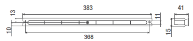
Aussenseite - Draufsicht
